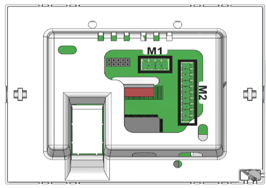
Achterzijde Smart WEB / EASY
